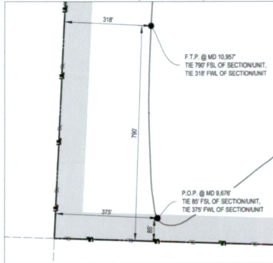
INSET "A" (NOT TO SCALE)
