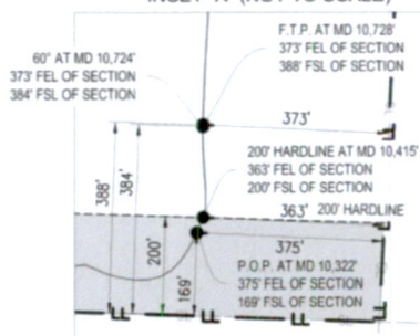
INSET "A" (NOT TO SCALE)
