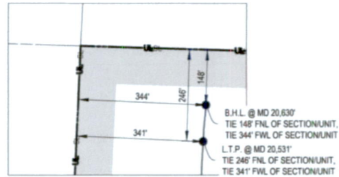
INSET "A" (NOT TO SCALE)
